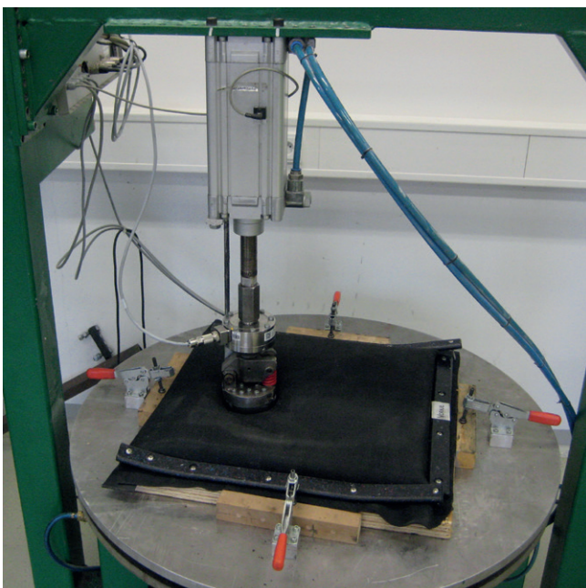
Bild 3: Dauertrittbelastung
